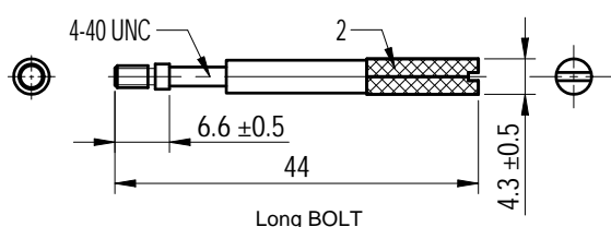
Long BOLT
